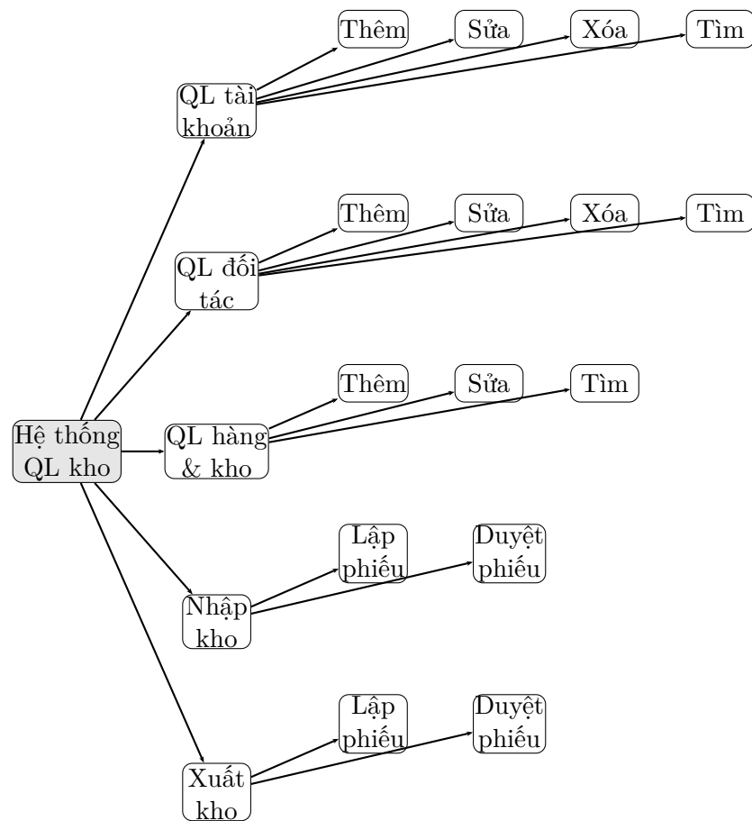
Figure 1: BFD: cấp 1 = nghiệp vụ chung; cấp 2 = hành động (use case)
